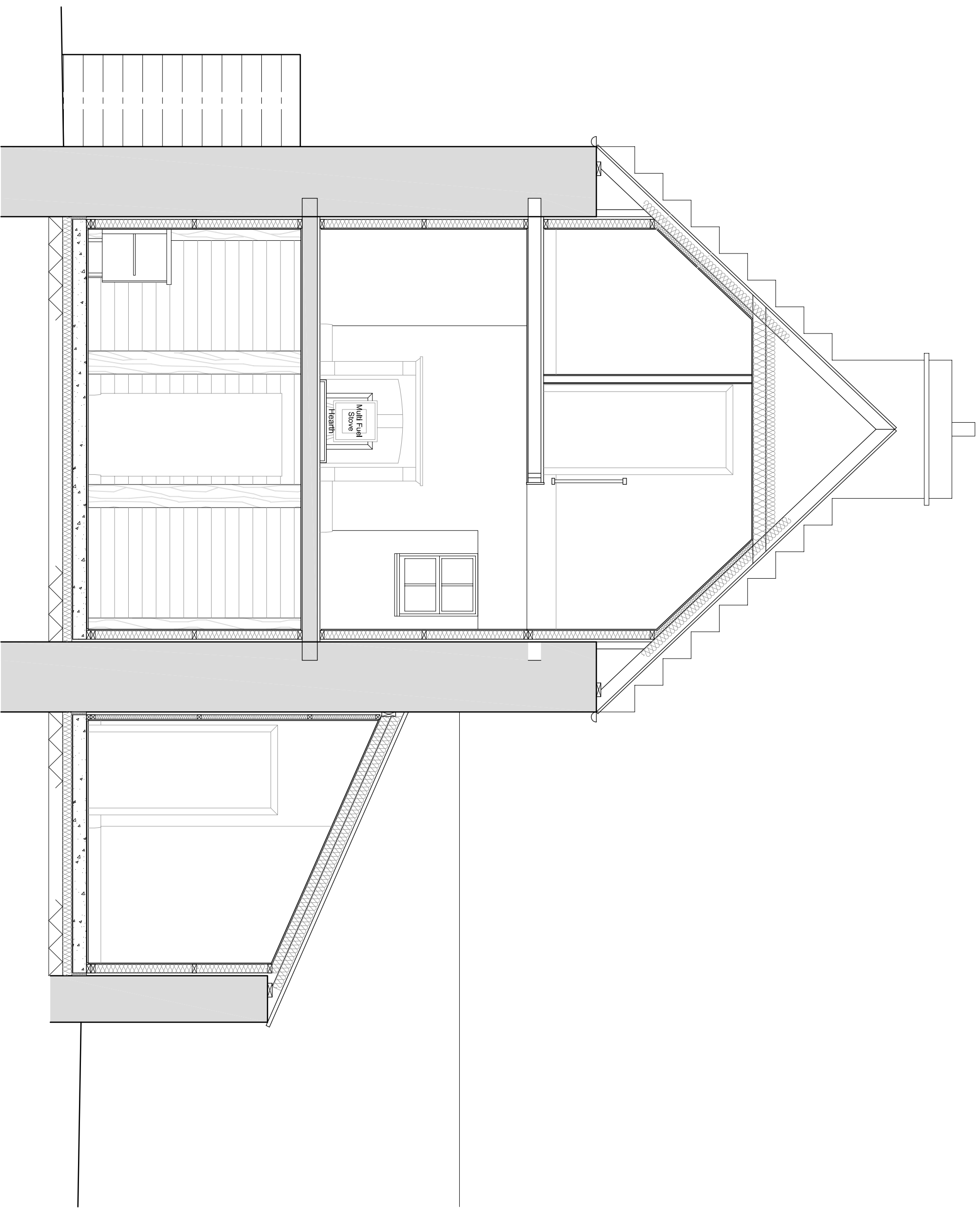
Section A-A Scale 1:100
